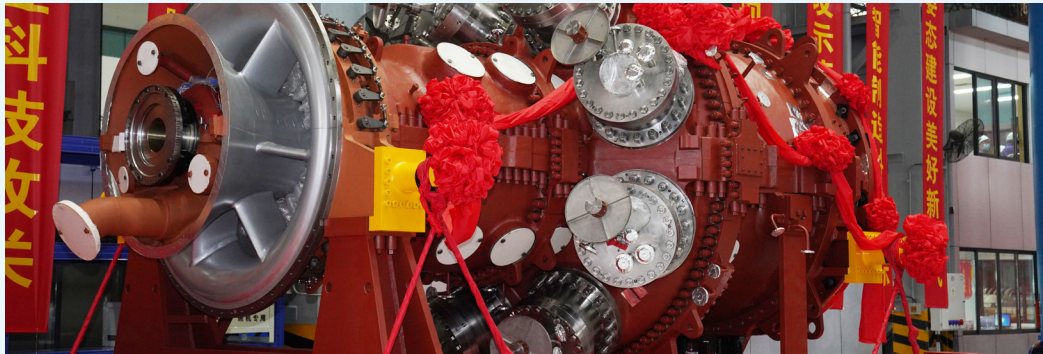
11月25日，国内首台完全自主知识产权的F级50兆瓦重型燃气轮机正式发运
